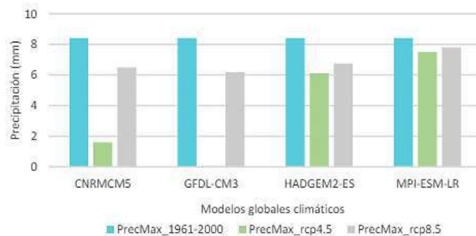
Figura 92: Comparativo de precipitación máxima del periodo 1961-2000 con proyecciones 2015-20239 del mes de septiembre con los cuatro MGC y con RCP 4.5 y 8.5
