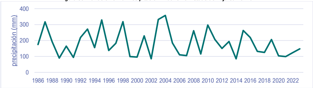
Cuadro 138. Promedio de precipitaciones
