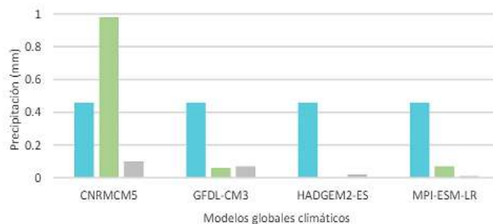
Figura 91: Comparativo de precipitación mínima del periodo 1961-2000 con proyecciones 2015-20239 del mes de junio con los cuatro MGC y con RCP 4.5 y 8.5
