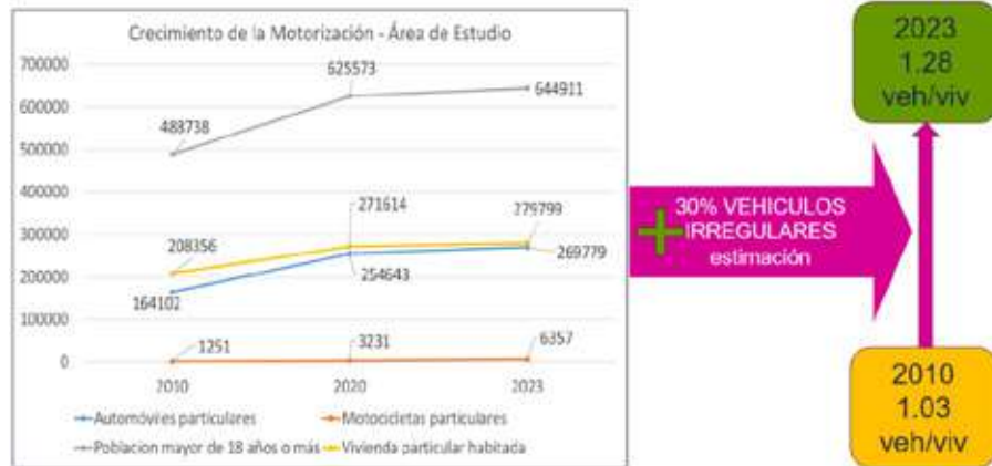
Figura 21. Crecimiento de la motorización área de estudio
