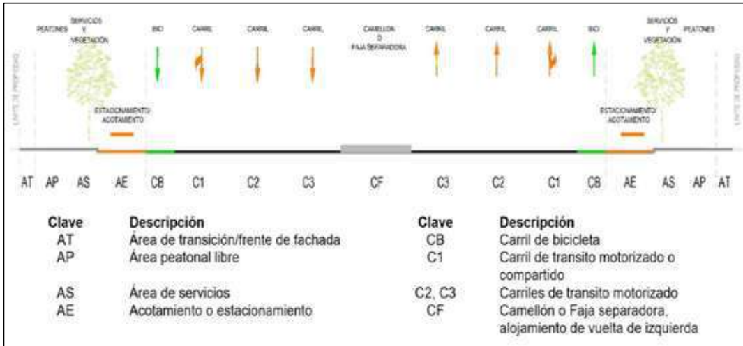
Figura 222: Componentes de la sección vial.
