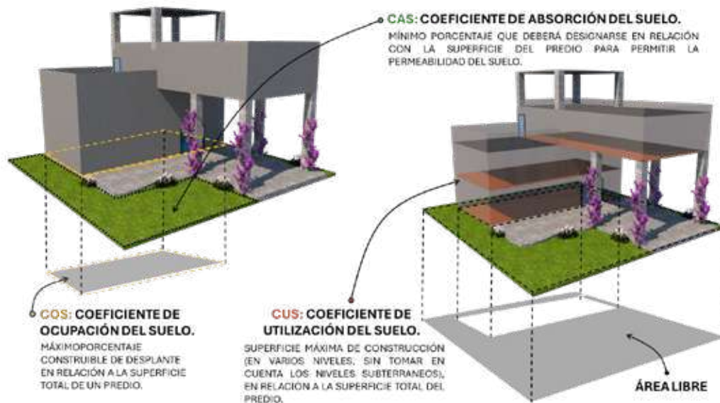
Figura 223: Coeficientes de regulación de la intensidad del suelo.
