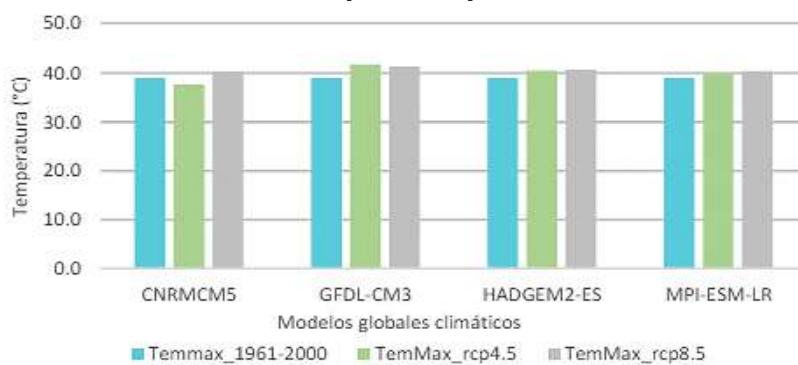
Figura 90: Comparativo de temperatura máxima del periodo 1961-2000 con proyecciones 2015-20239 del mes de enero con los cuatro MGC y con RCP 4.5 y 8.5
