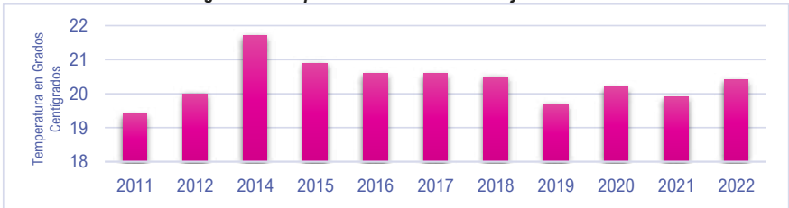
Figura 87. Temperatura Media Anual en Baja California
