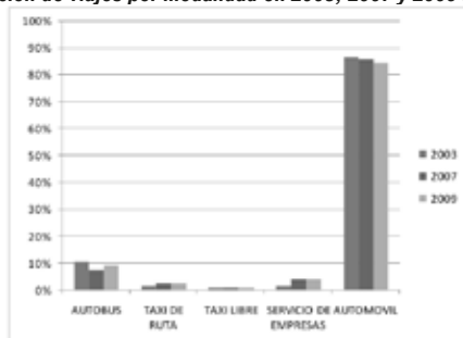
Figura 18. Distribución de viajes por modalidad en 2003, 2007 y 2009 reportada en PMVyT
